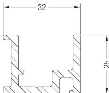
Направляющая ROTO INTELIO® SLIDE
