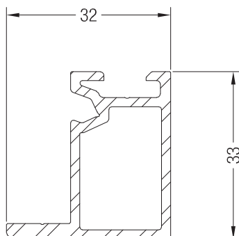
Притвор Houtau INTELIO® SLIDE
