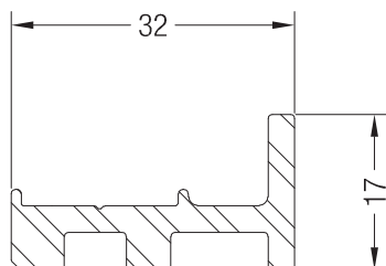
Притвор ROTO INTELIO® SLIDE
