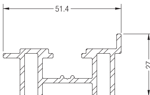
Адаптер ROTO INTELIO® SLIDE
