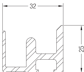
Опорная шина Houtau INTELIO® SLIDE
