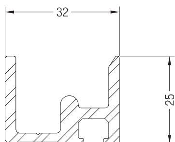
Опорная шина ROTO INTELIO® SLIDE
